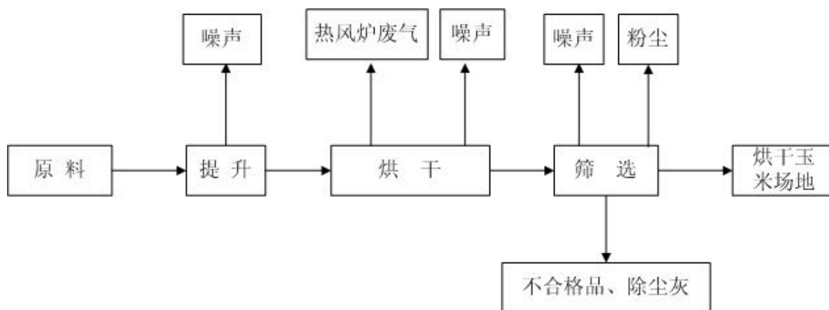
图 4 生产线工艺流程示意图
